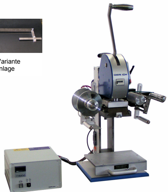
Ausführung der P-800 mit einem Dekorfolienvorschub
